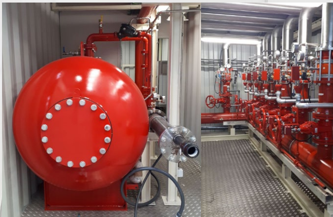
Überflutungsventile mit TRIM-Steuerung. Foamogen-Mischzentrum.
